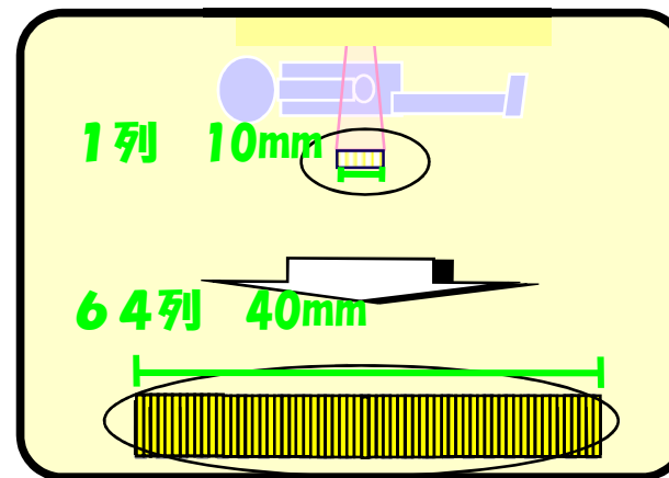
図2 検出器の拡大図
